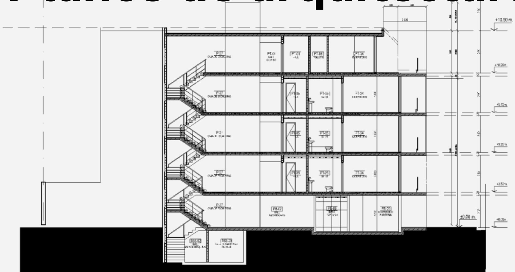
CORTE B-B
