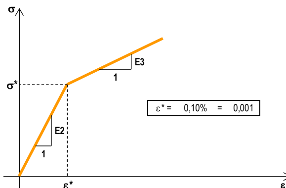
RELACIÓN "2" \sigma = f(\epsilon)
