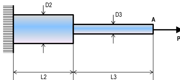
ESQUEMA ESTRUCTURAL "B"
