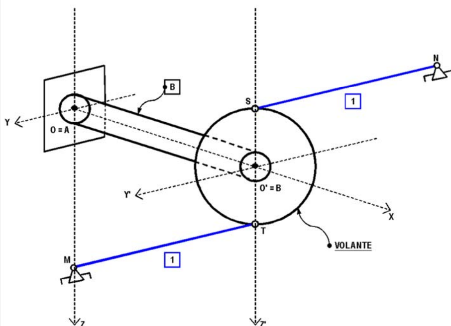
EJERCICIO N° 05 - FIGURA N° 05.03: VISTA AXONOMÉTRICA
