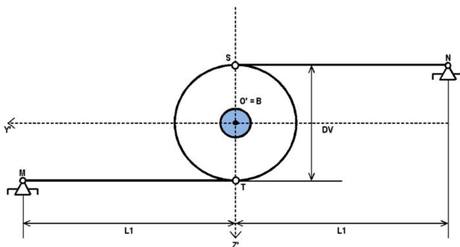
EJERCICIO N° 05 - FIGURA N° 05.02: VISTA FRONTAL
