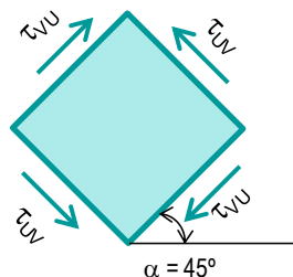
TERNA (O;U;V;W)
